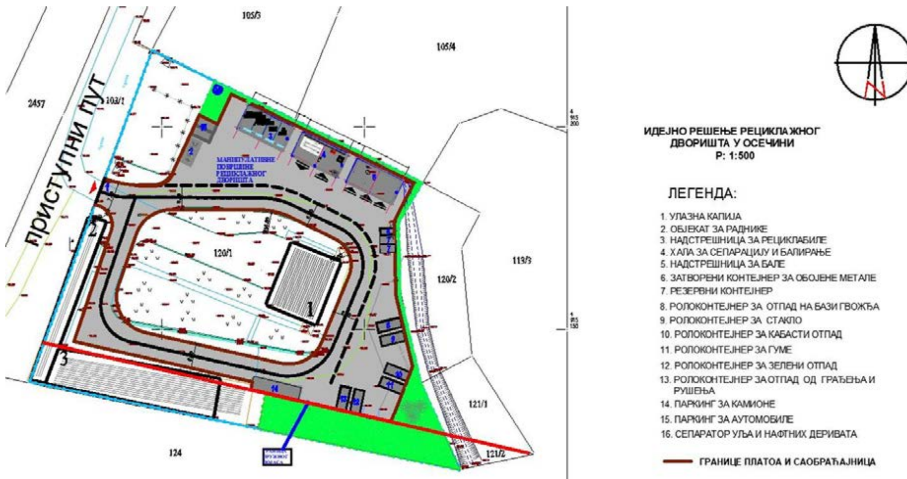
Слика 17.7.1-1. Ситуациони план Рециклажног дворишта у Осечини (Извор ИДР, ЦИП и “ИНСТИТУТ WALTER KOCH” 2023. године)
