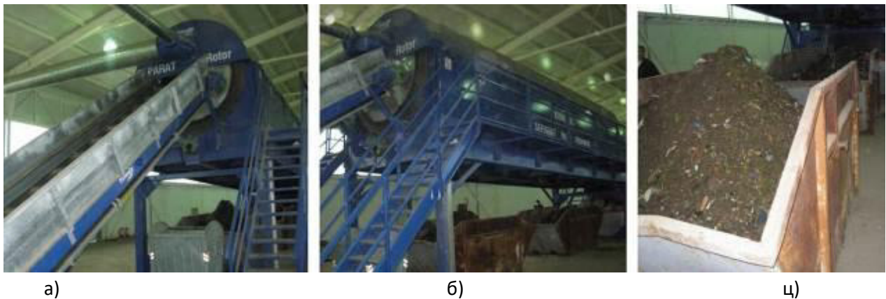
Слика 4.6.3-6. Рото сито а) Подизна оребрена трака на улазу у рото-сито; б) рото-сито; ц) биоразградиви отпад у контејнерима, смештеним испод рото-сита
