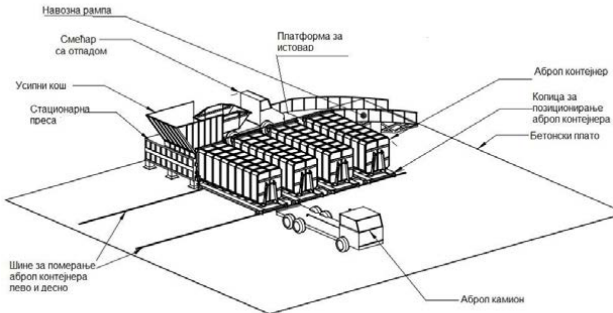
Слика 17.2.1-1. Елементи аутоматске претоварне станице са сабијањем отпада
