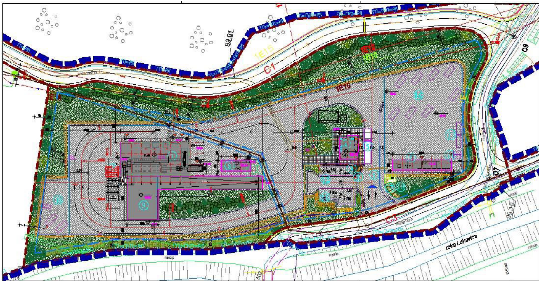
Слика 17.12.1-2. Ситуациони план комплекса ТРСЦ у Лазаревцу (Извор ПГД, ЦИП, СЕТ и ИНСТИТУТ WALTER KOCH 2023. године)
