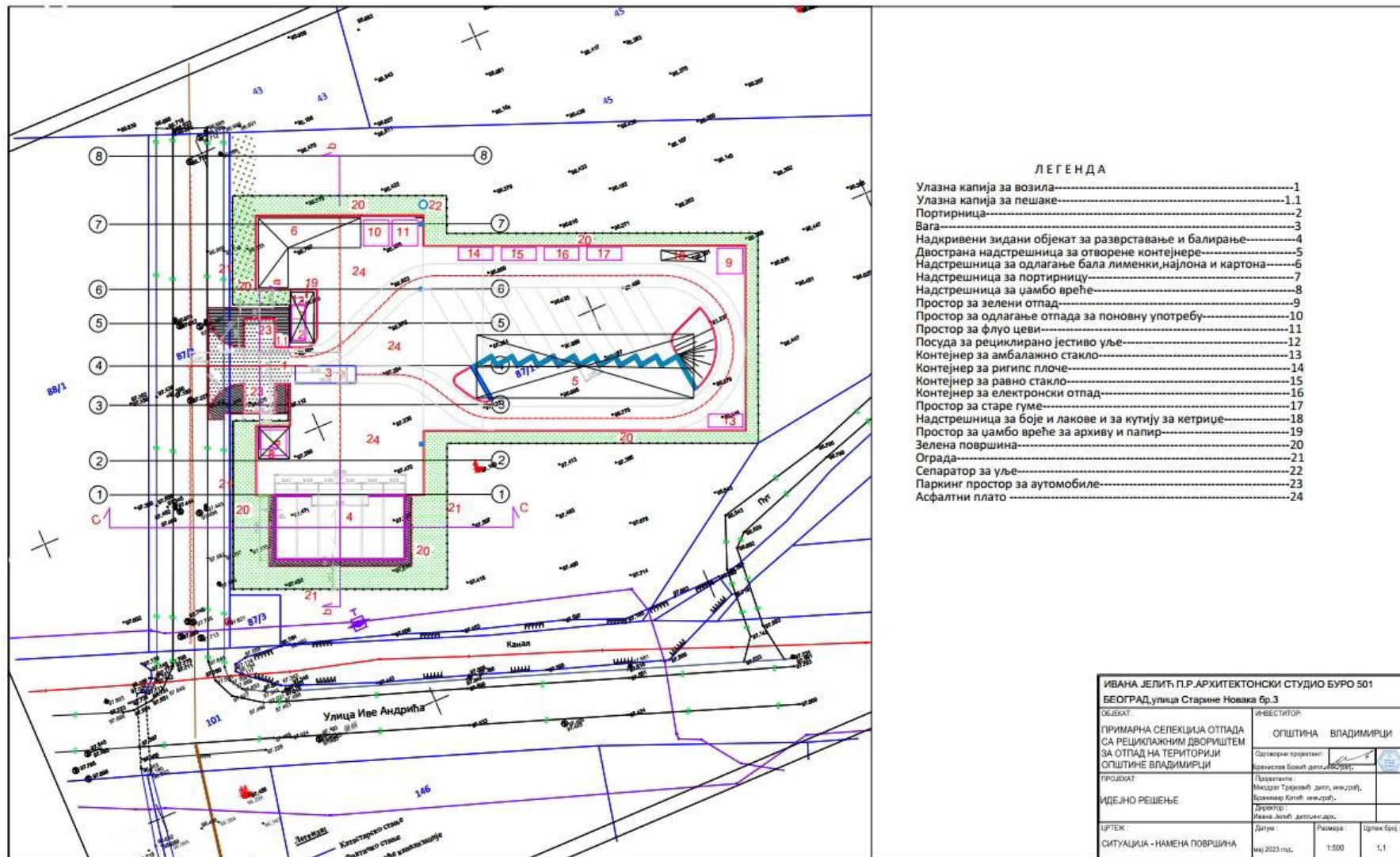
Слика 17.8-1. Ситуациони приказ концептуалног решења центра за сакупљање отпада на подручју општине Владимирци (Извор ИДР, Ivana Jelić PR Arhitektonski studio BURO 2023. године)
