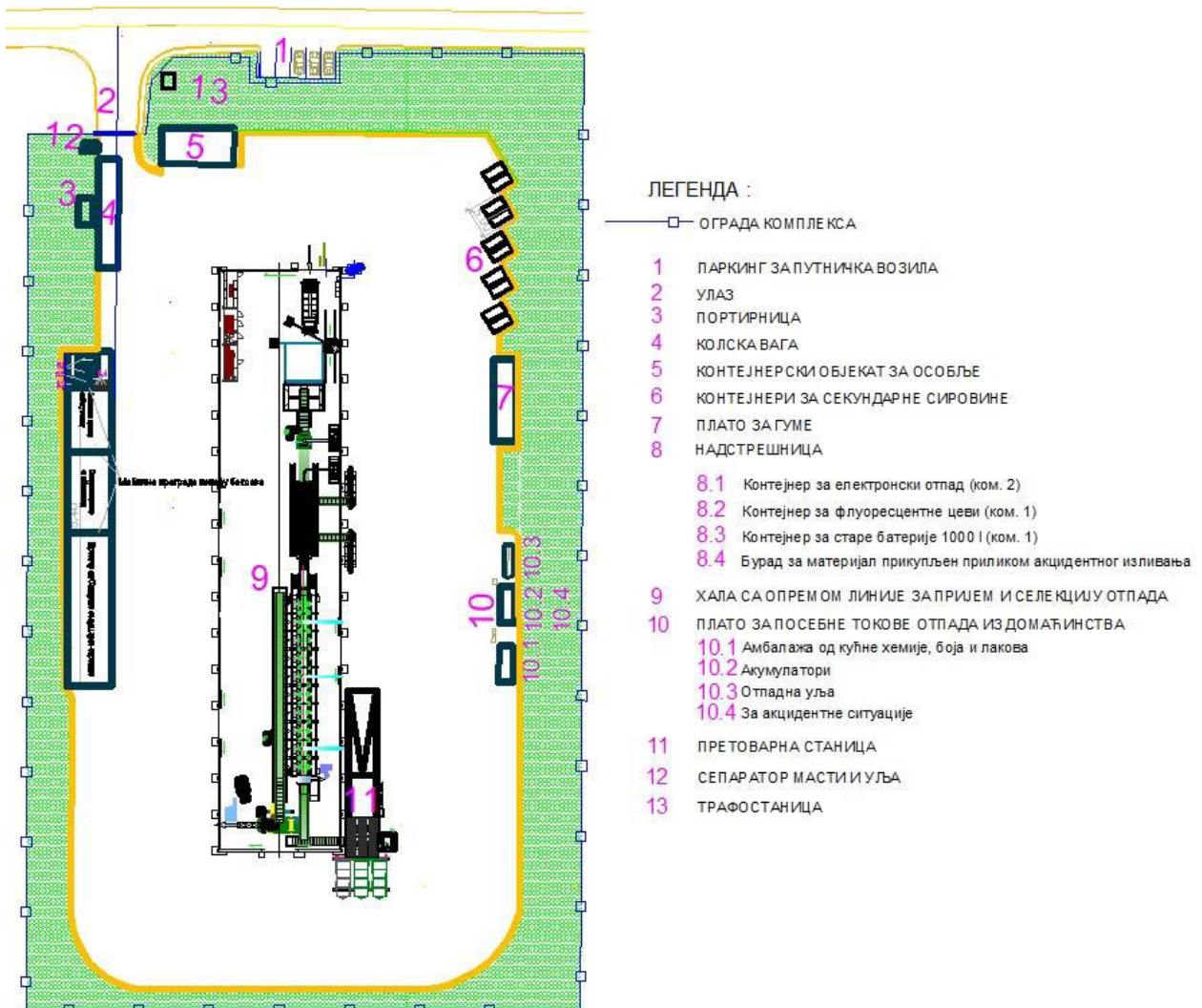
Слика 17.14-2. Распоред објеката и опреме на ТС са селекцијом отпада - идејни концепт
