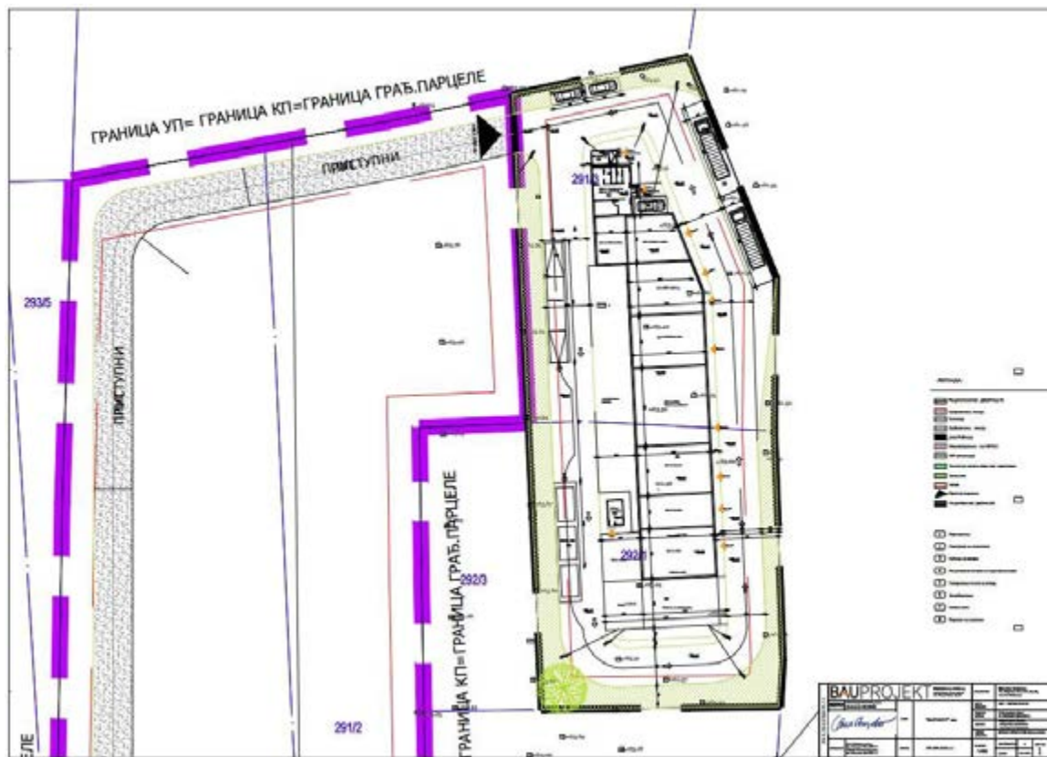
Слика 17.6.1-1. Ситуациони план рециклажног дворишта у Мионица селу (Извор ИДР, Баuproјект 2023. године)
